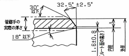
ベベルエンドの形状・寸法
