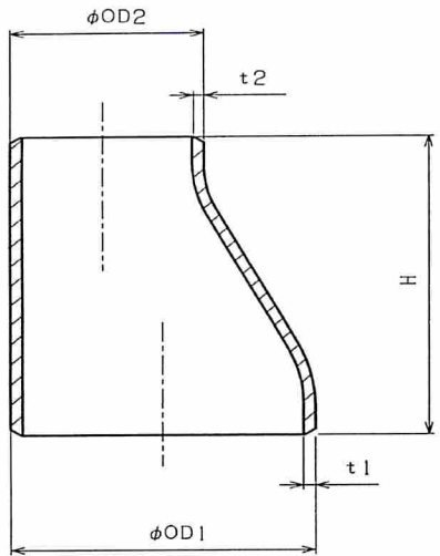
偏心レジューサ
