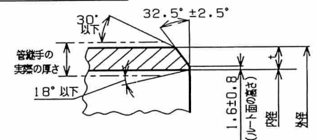
ベベルエンドの形状・寸法
