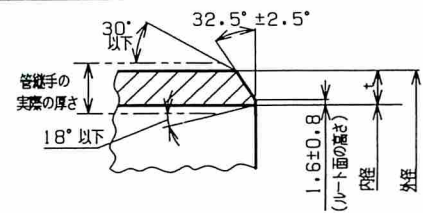
ベベルエンドの形状・寸法
