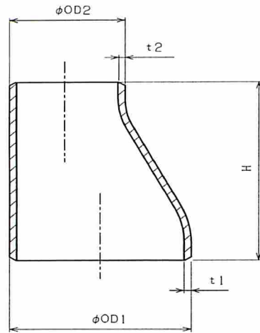
偏心レギュレーサ
