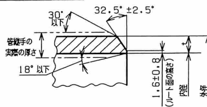
ベベルエンドの形状・寸法
