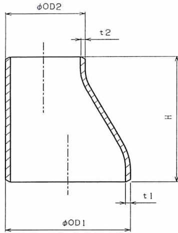
偏心レジュューサ
