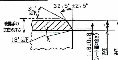
ベベルエンドの形状・寸法
