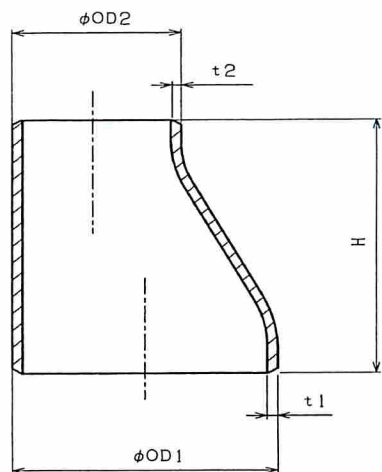
偏心レジャーサ
