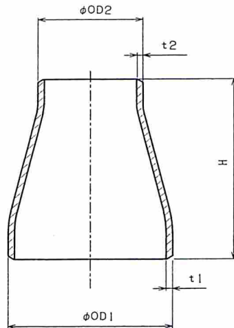
同心レジューサ
