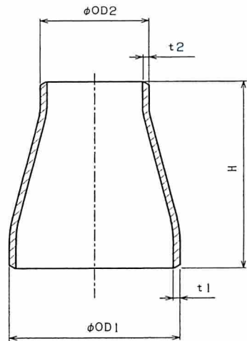
同心レギュレーサ
