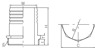
捻込型ホースニップル
