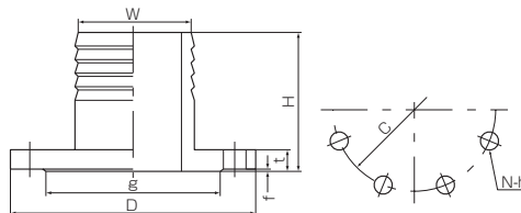
10K フランジ型ホースニップル
