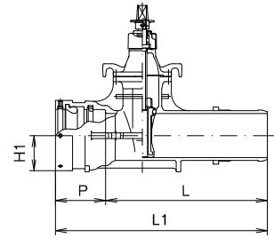
NSソフト (内ねじ式・受挿し形)
