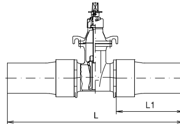
ポリパイソフト(内ねじ式・両袖管形)
