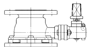
呼び径 75mm×面間150mm
