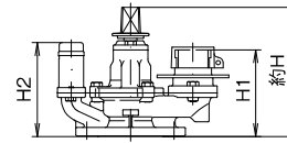
ステンレス製消火栓 排気弁付 単口75
