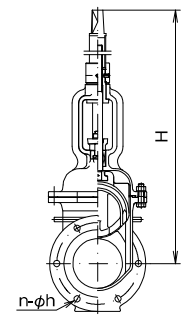
ニューボブ (外ねじ式・キャップ式)
