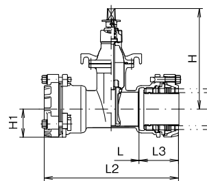
PE-NOVO形ソフト (内ねじ式)
