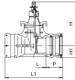
NSソフト (内ねじ式・両受形)
