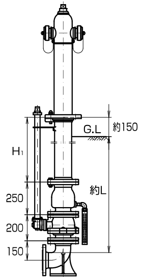
呼び径100mm II型 回転打倒式 補修弁・乙管付
