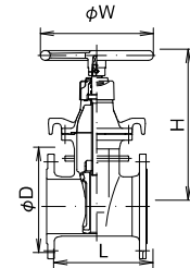
ソフトシール仕切弁 (内ねじ式・ハンドル車式)
