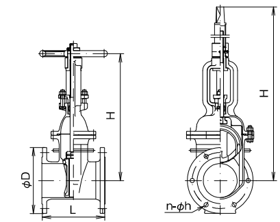
ニューボブ (外ねじ式・ハンドル車式)
