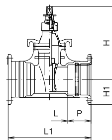
GXソフト (内ねじ式・両受形)
