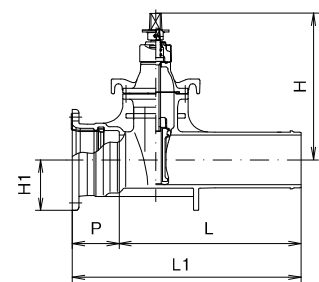
GXソフト (内ねじ式・受挿し形)
