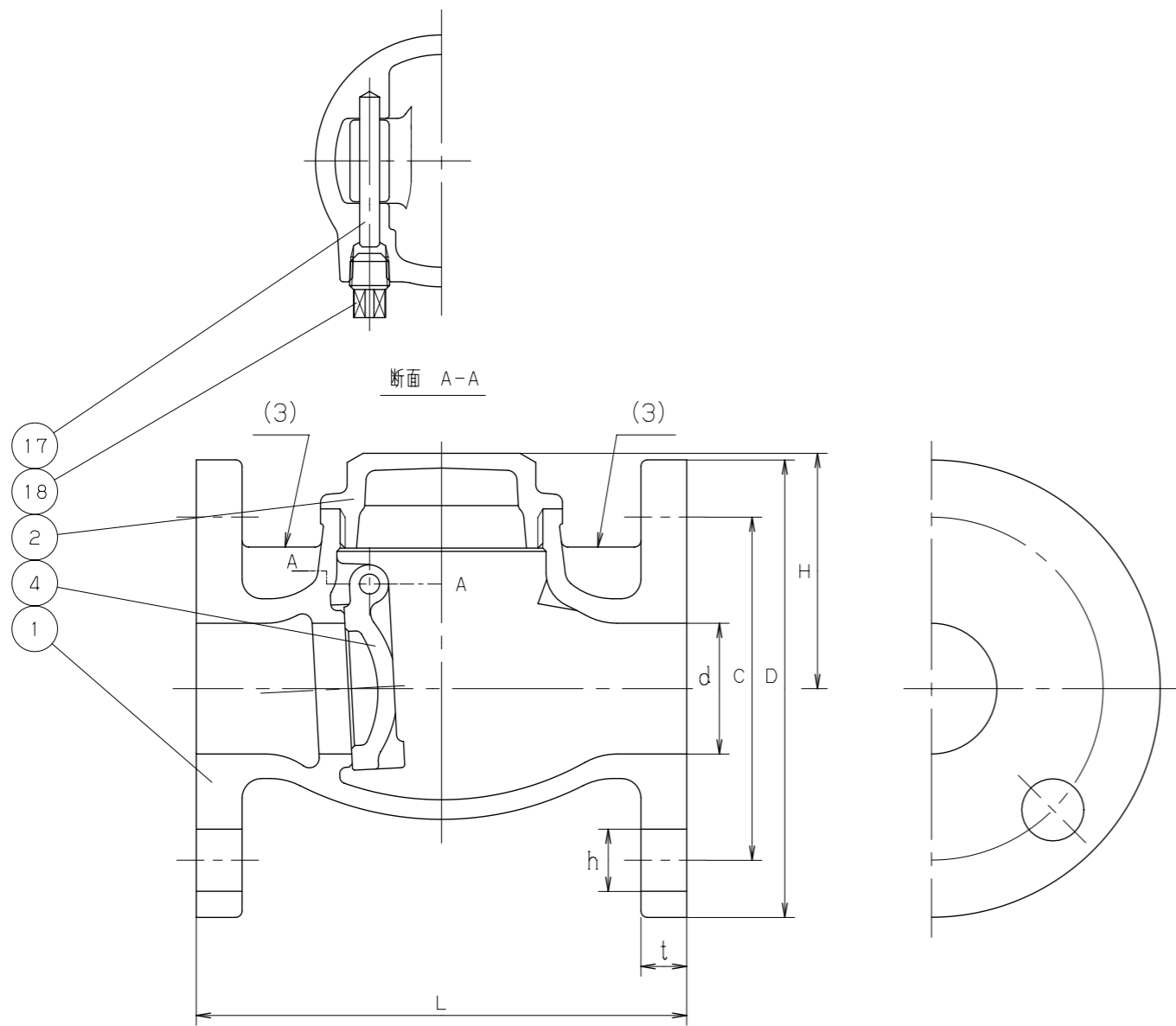
寸法表
