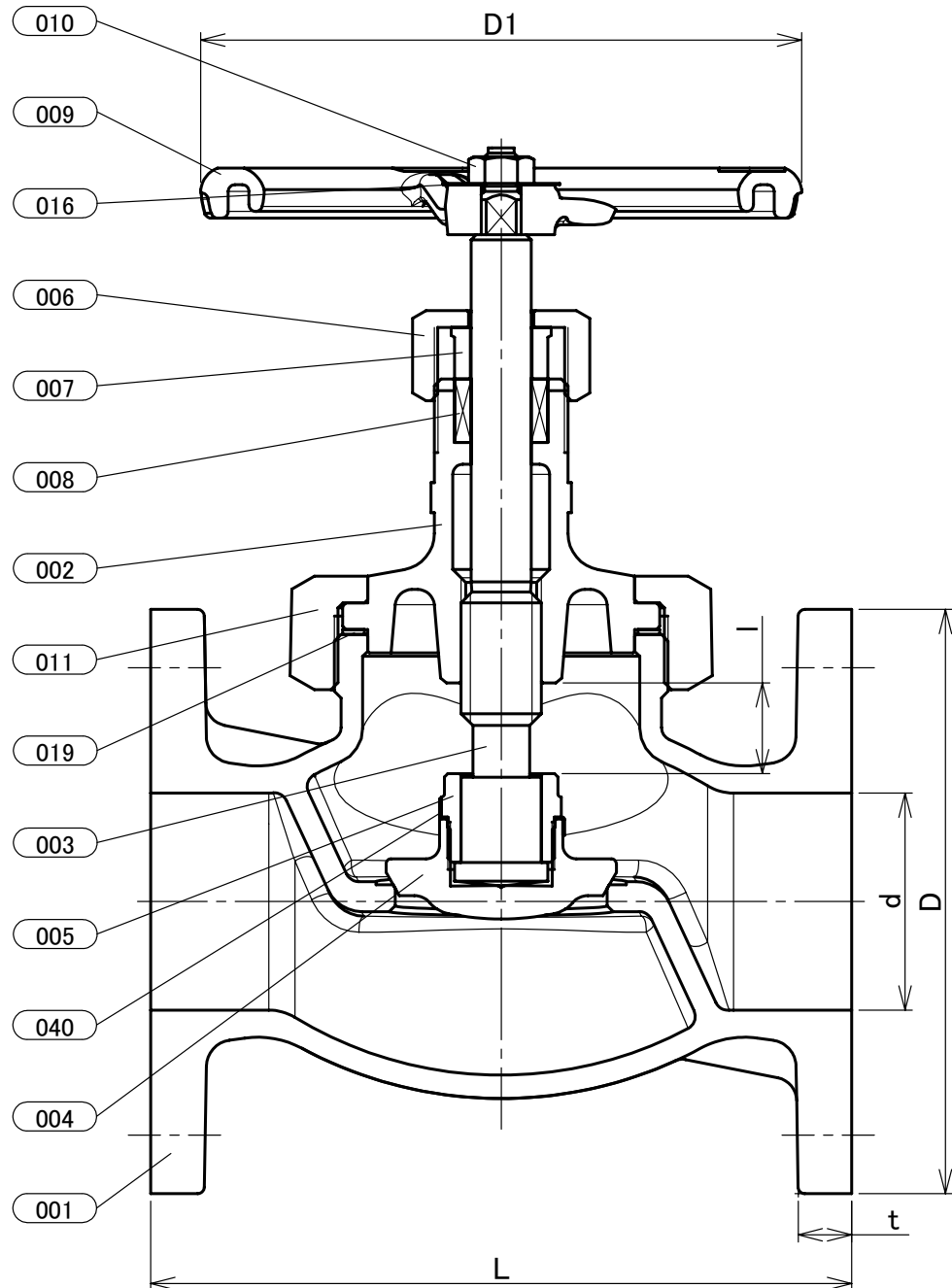
寸法表
