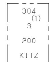
鑄出し表示
