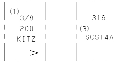
呼び径 3/8 のみ
