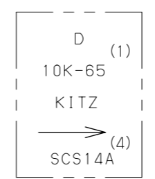
呼び径 65&80 鑄出し表示
