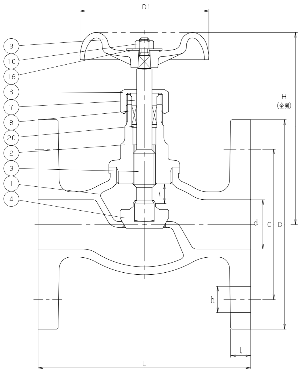
寸法表
