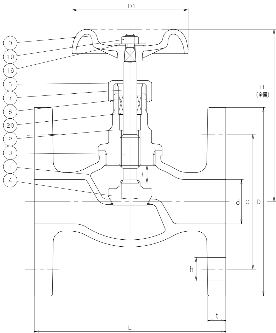
寸法表
