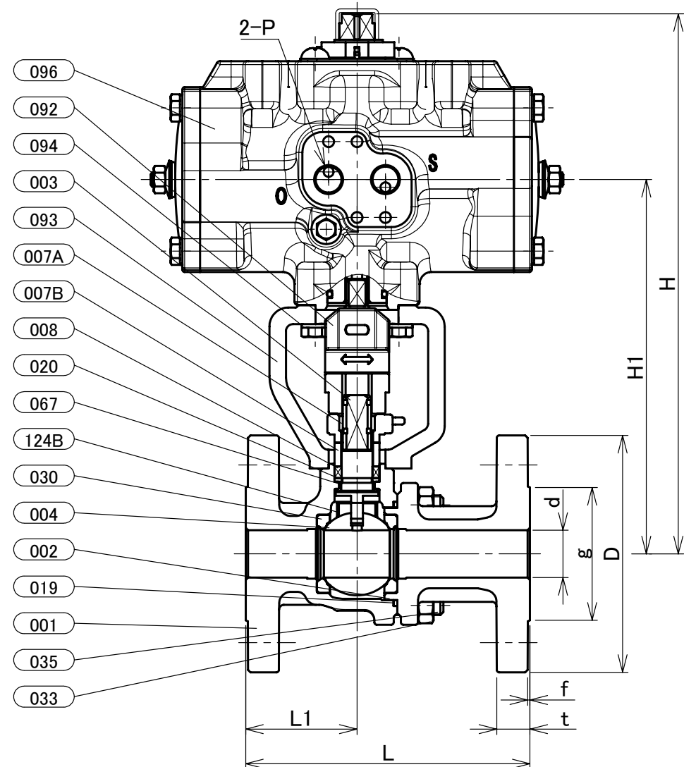
寸法表
