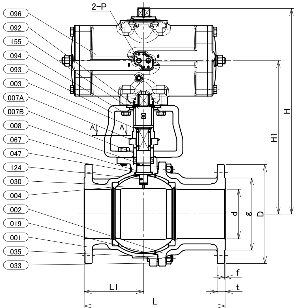
寸法表
