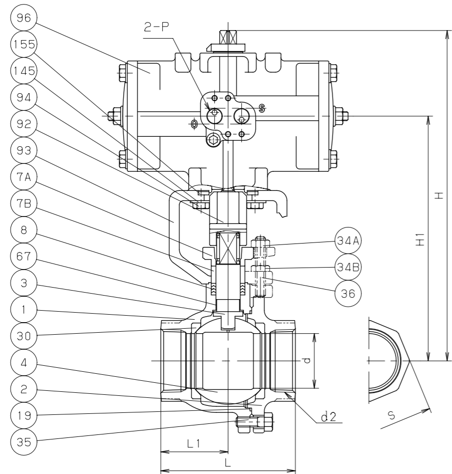
寸法表
