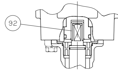
呼び径 50-65, 125-200
