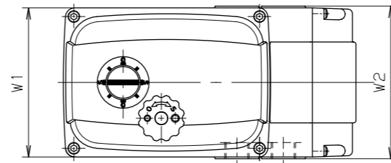
矢視 A
