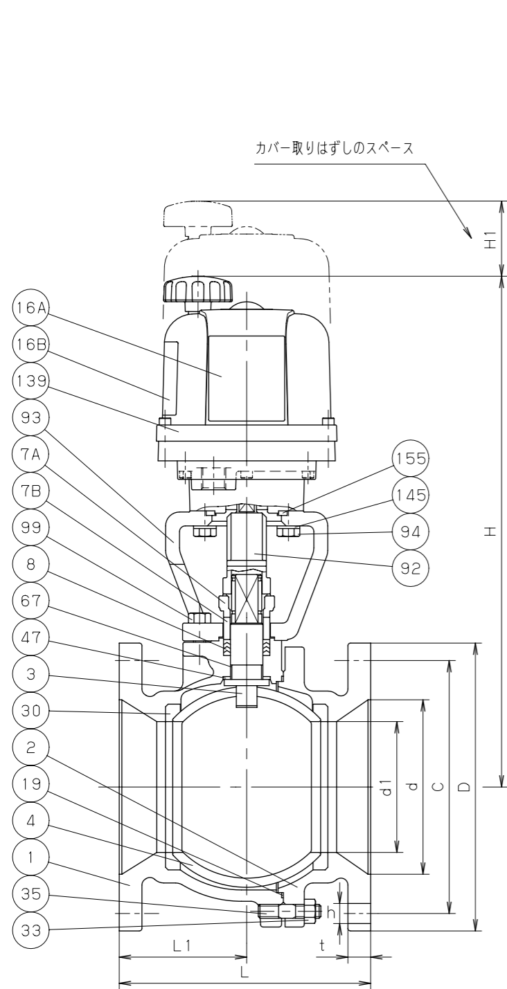
寸法表
