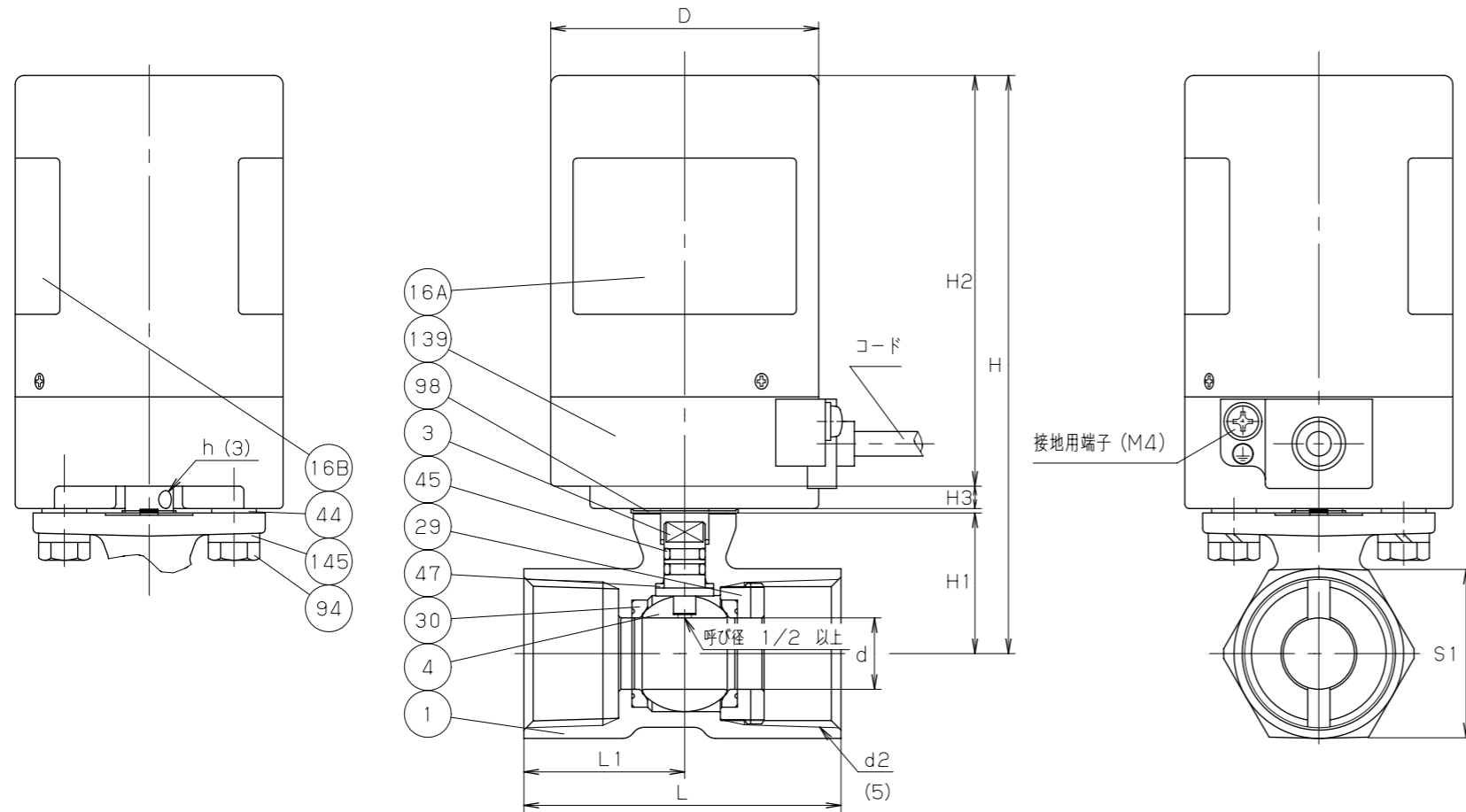
寸法表
