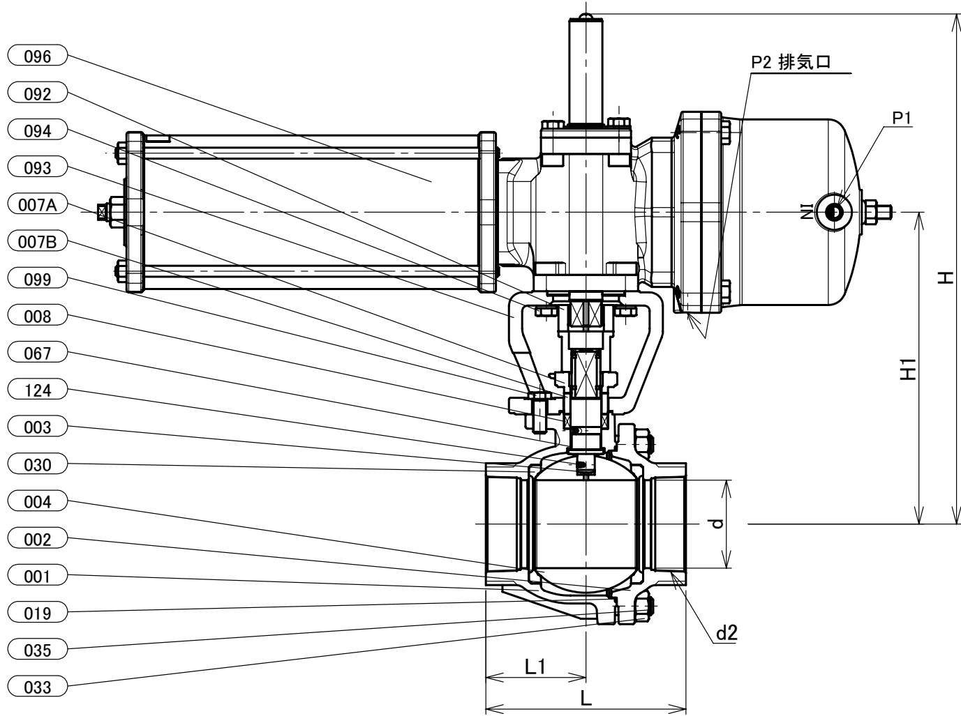
寸法表
