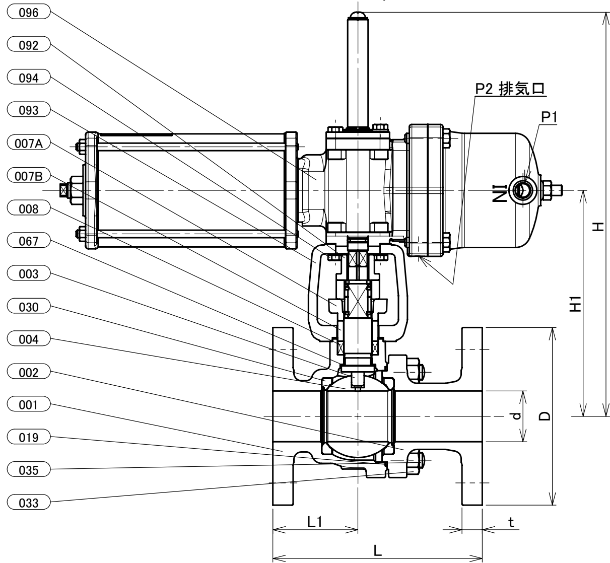
寸法表
