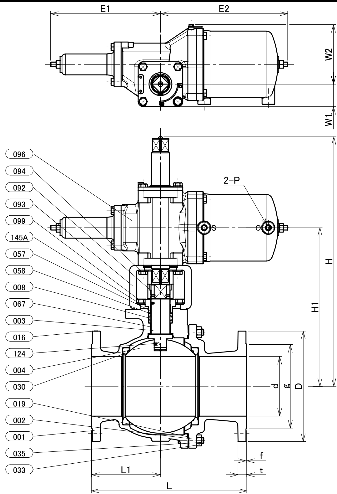
寸法表
