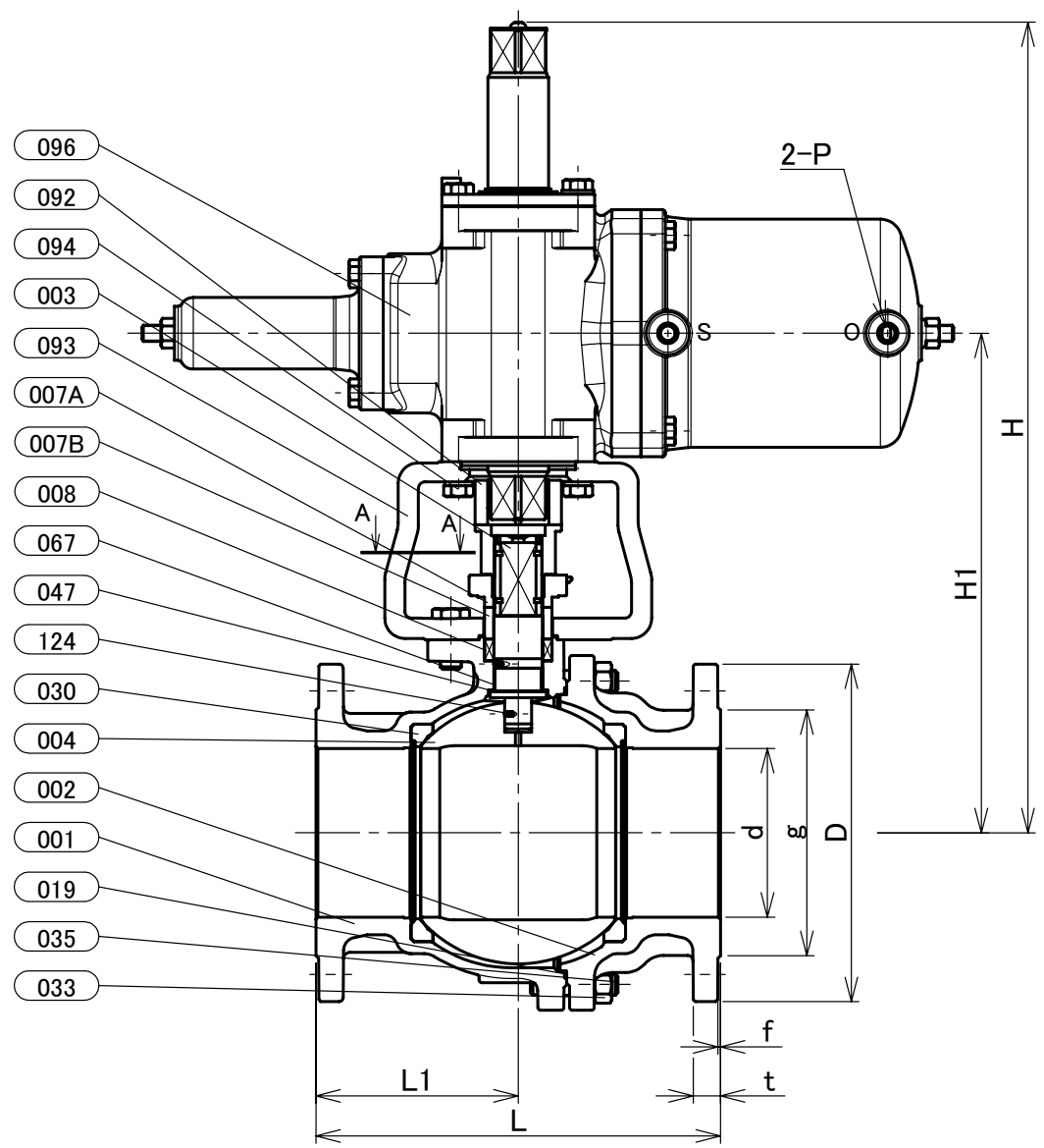
寸法表
