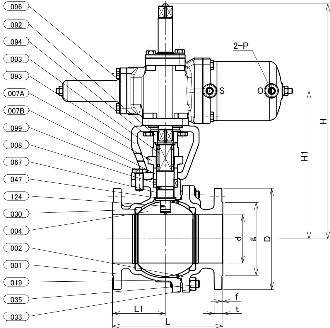
寸法表
