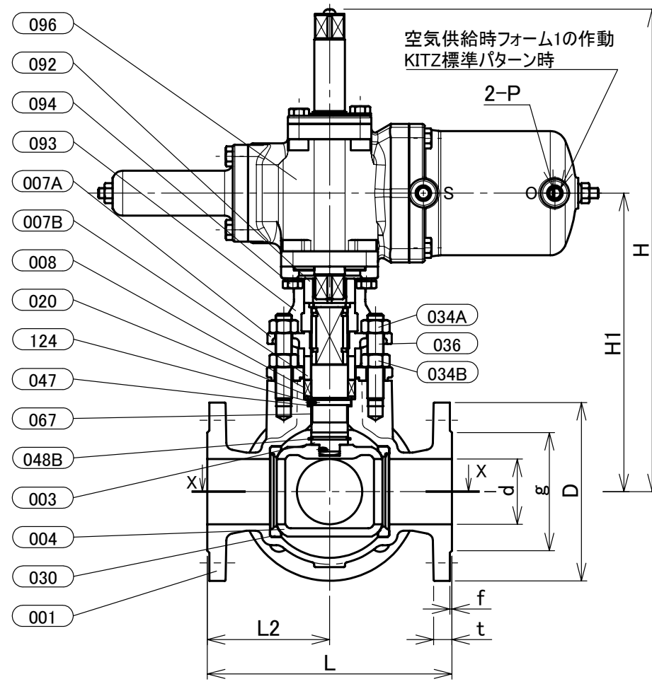
寸法表
