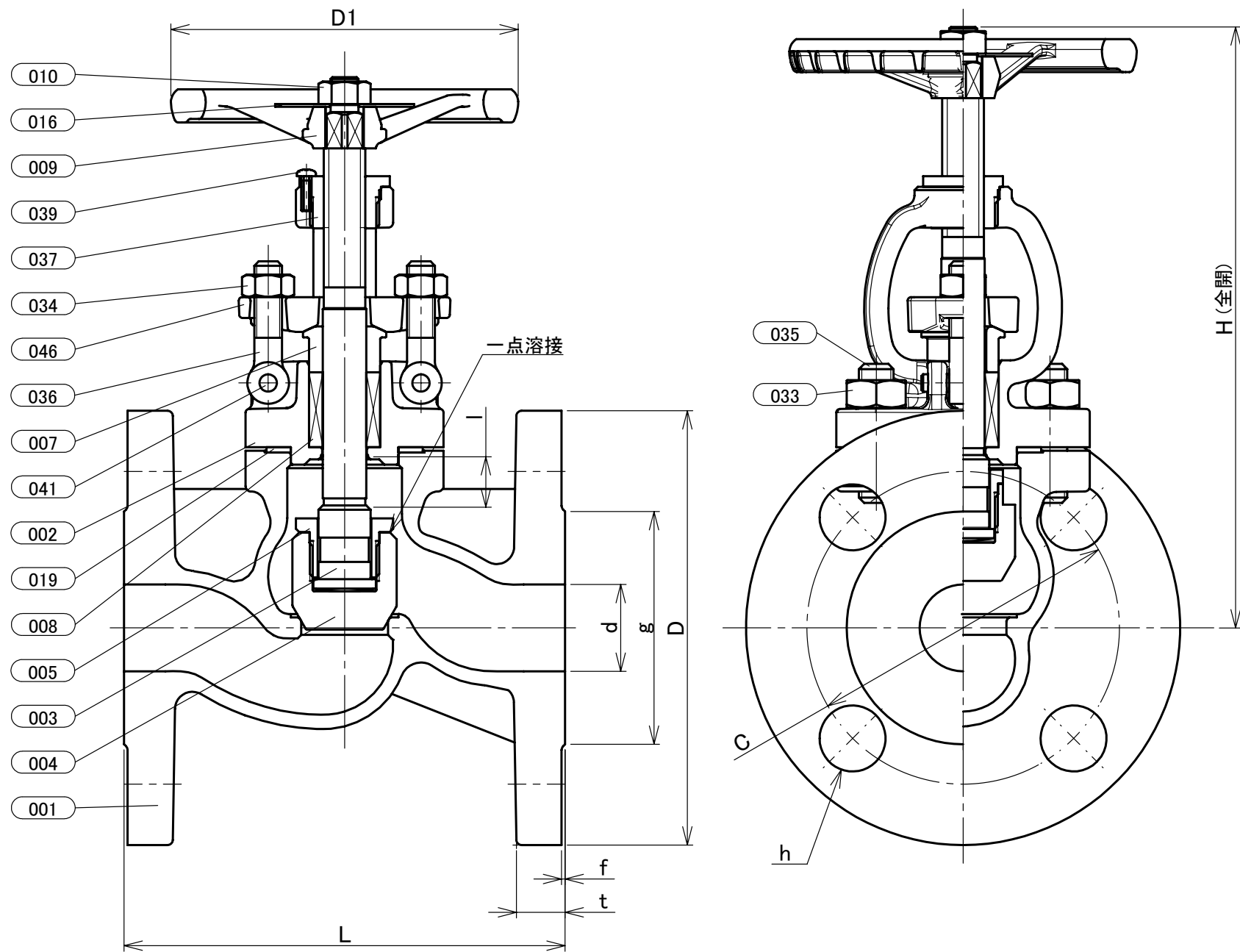
寸法表
