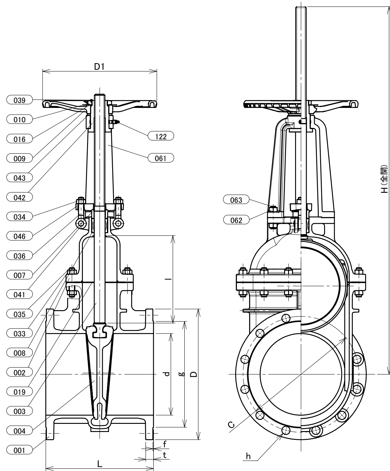
寸法表 単位:mm
