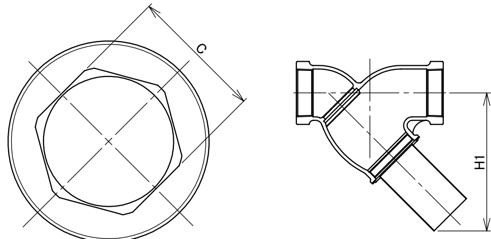
矢視A
