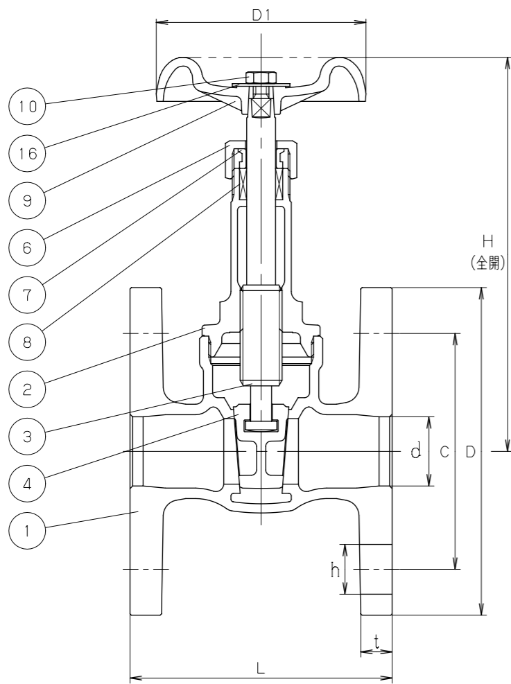
寸法表
