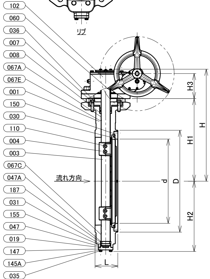
寸法表
