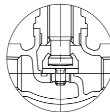
呼び径 1/4 のみ
