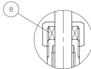
呼び径 1/4&3/8
