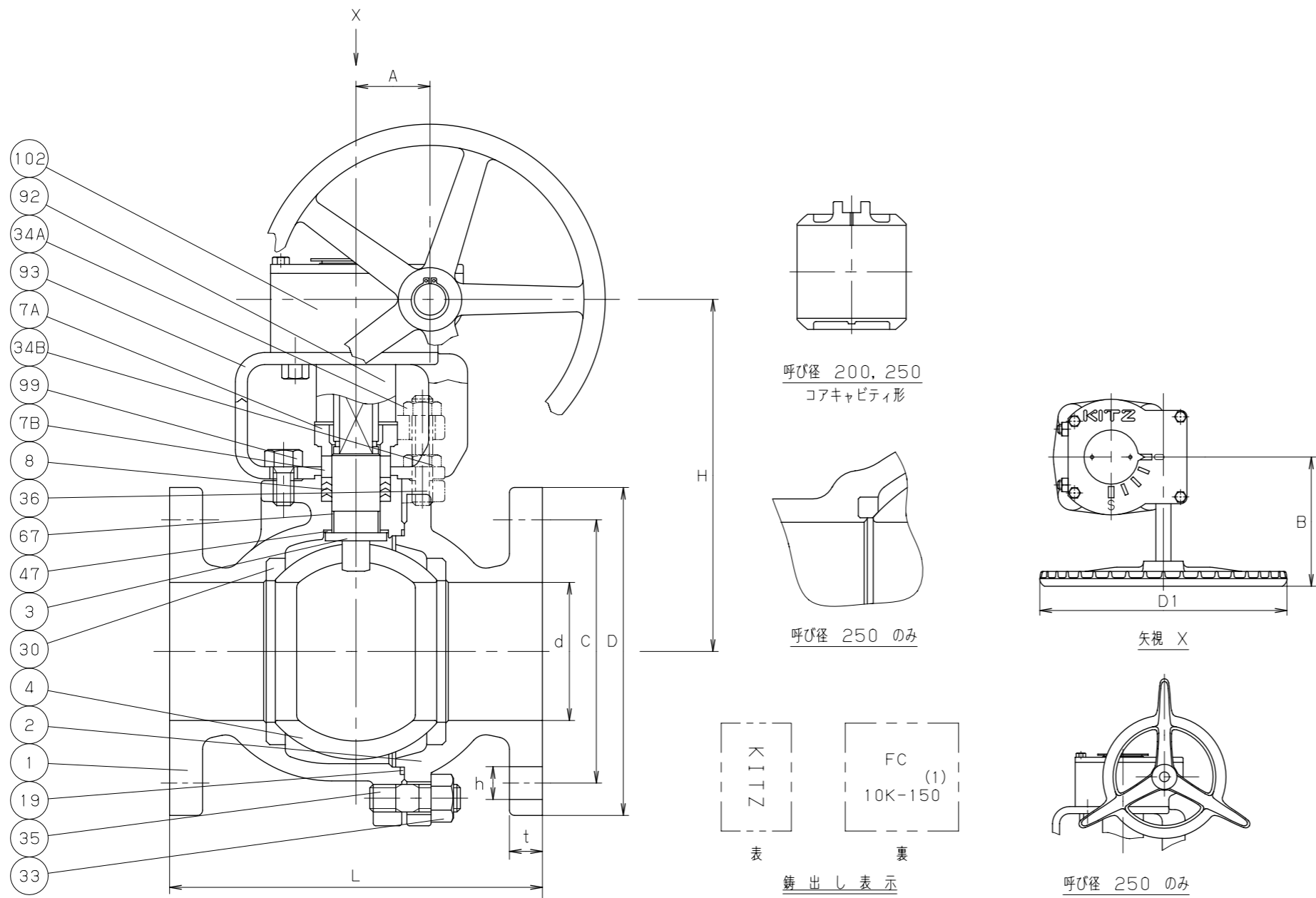
寸法表
