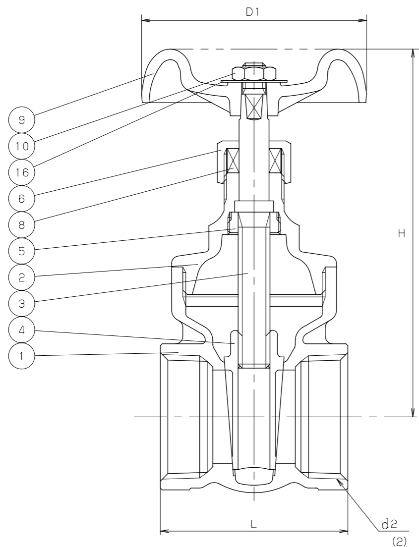
寸法表
