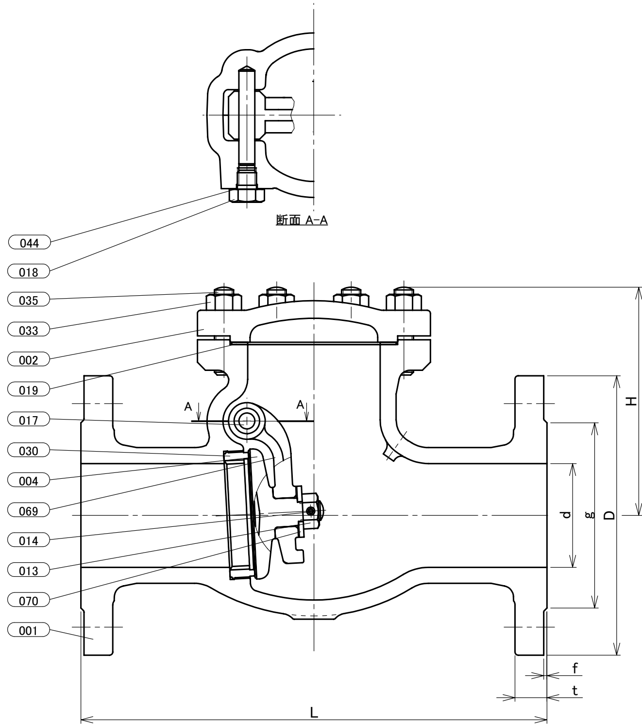
寸法表
