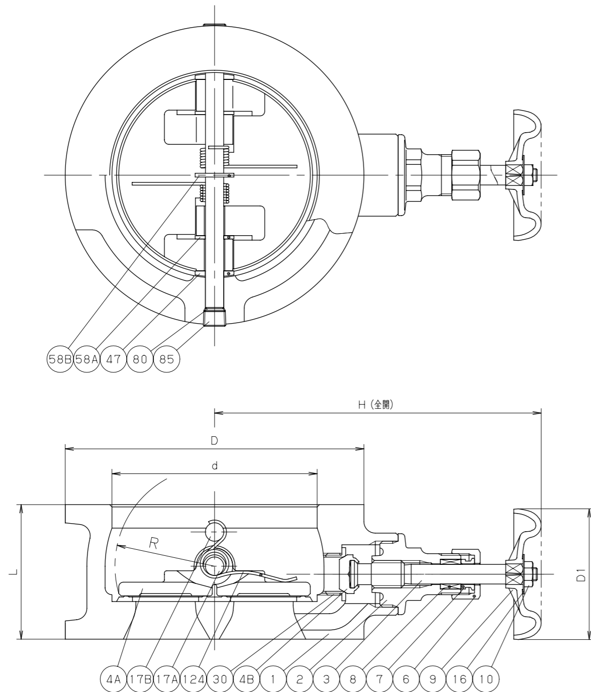
寸法表
