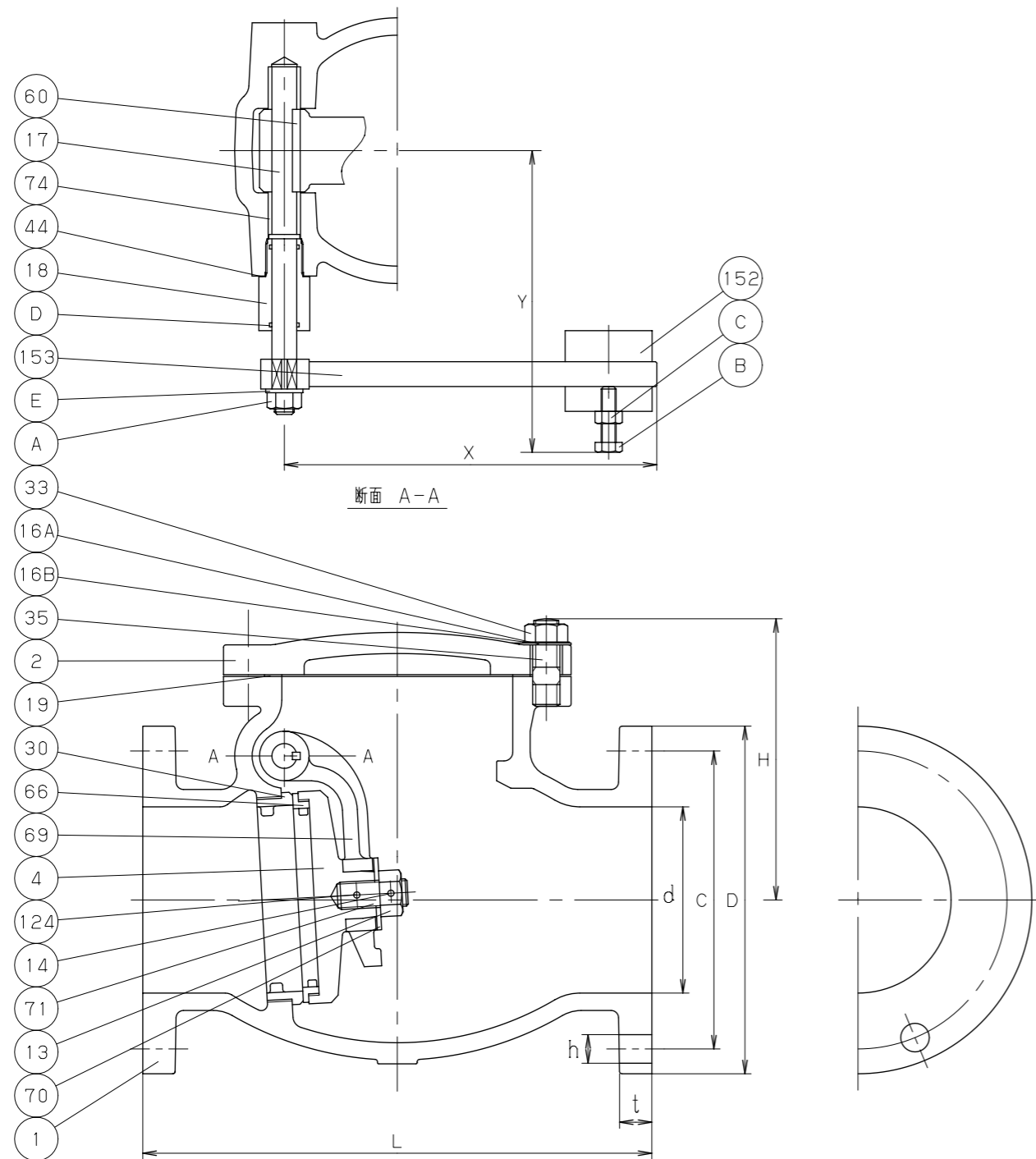
寸法表
