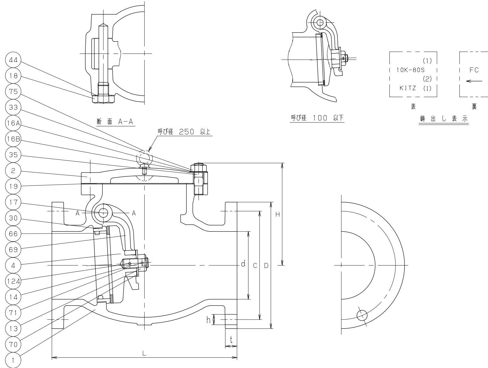
寸法表
