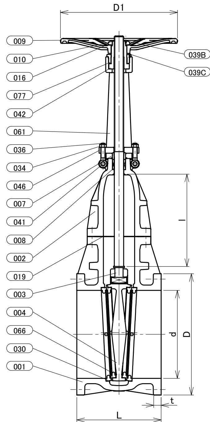
寸法表
