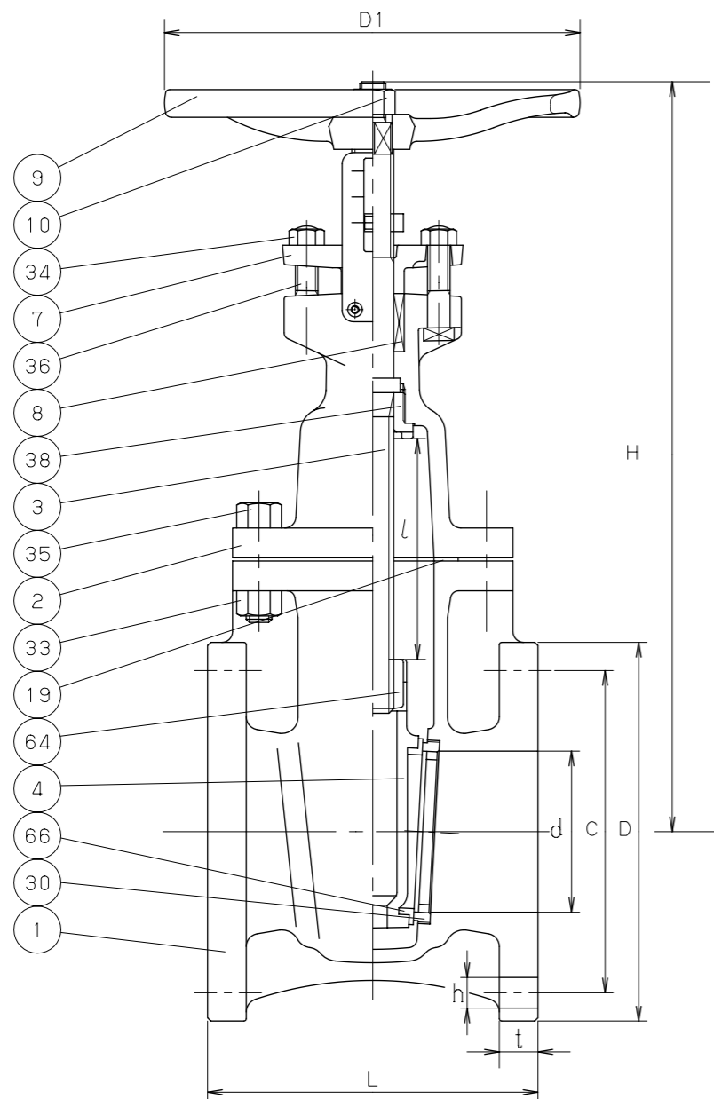
寸法表
